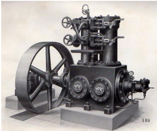
Stehender Gleichstrom-Kompressor mit schmiedeeisernem Kurbelgehäuse
