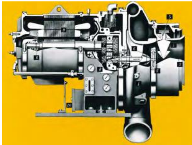
Hermetischer Turboverdichter 19DA Carrier
