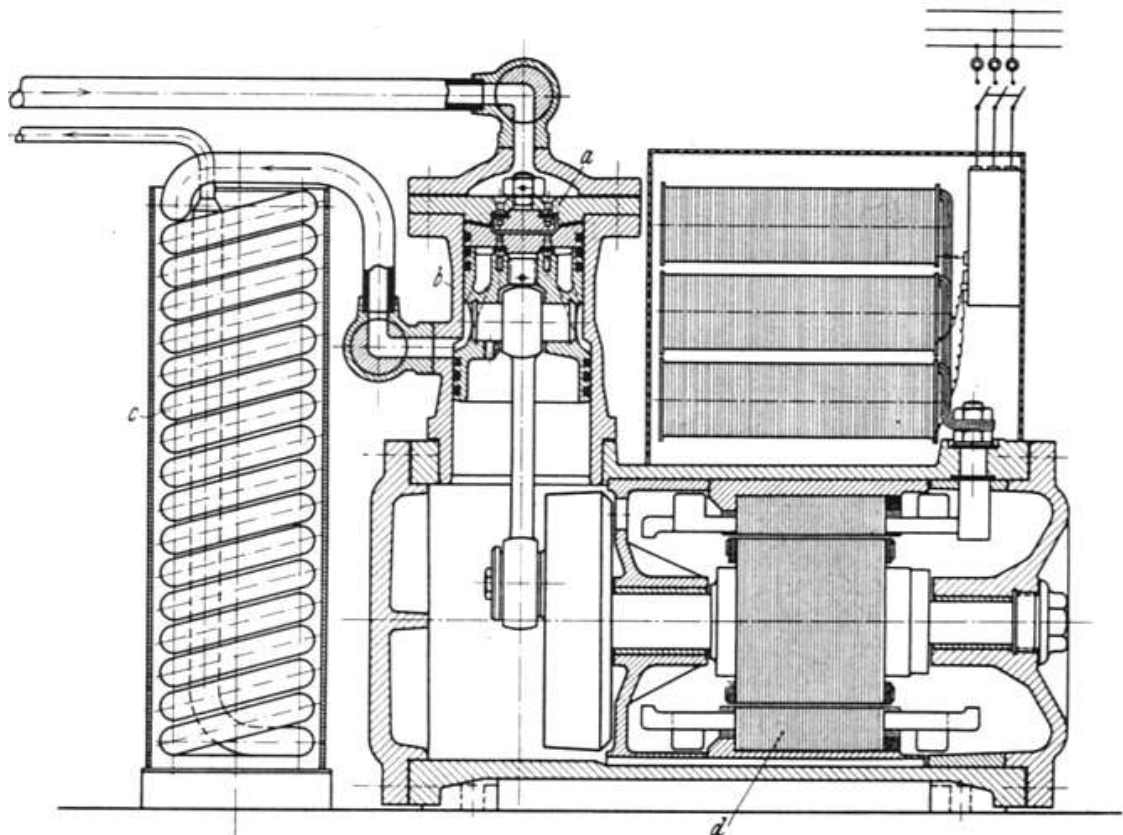
Stopfbuchsloser Ammoniakverdichter (Freundlich). a Saugventil, b Druckventil, c Verflüssiger, d Motor.
