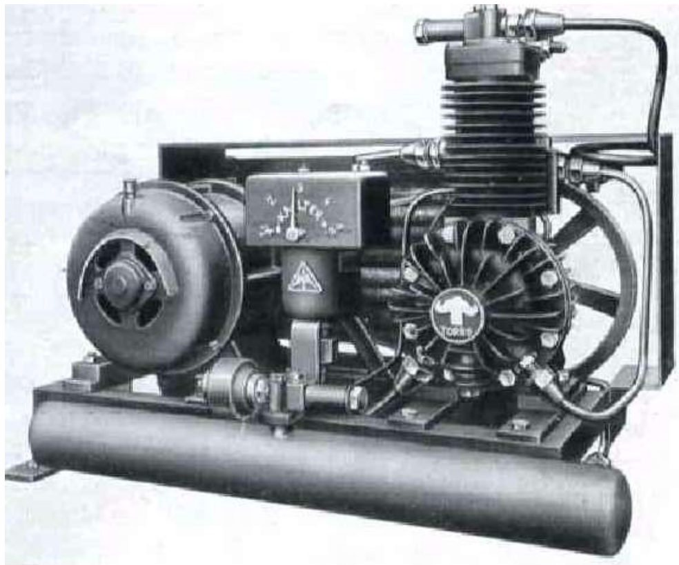
„Torro“-Kälteautomat, luftgekühlt, 1190 Kcal/h.
