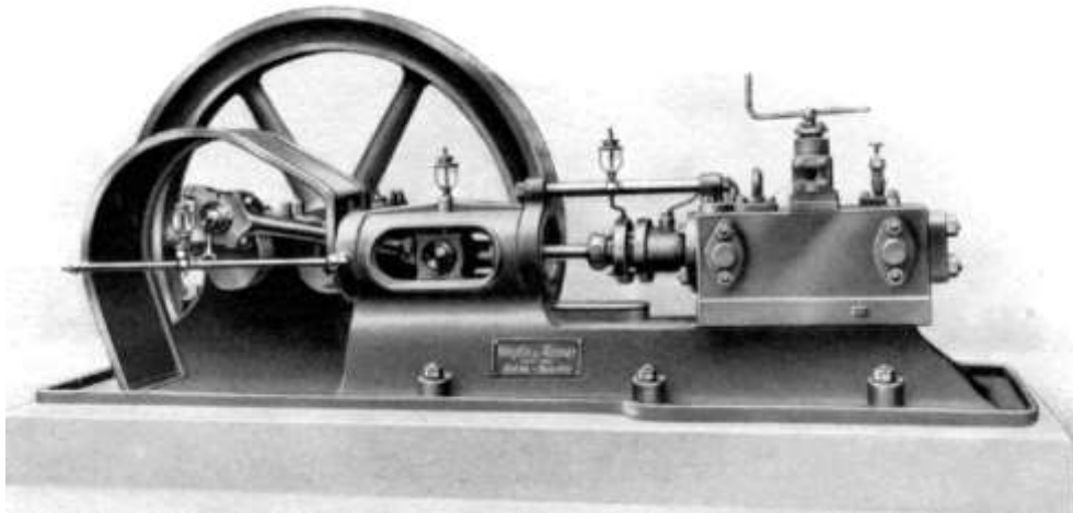
CO 2 Verdichter von Wegelin & Hübner um 1900
